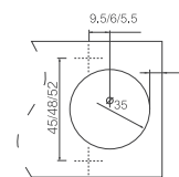
Hole Size 钻孔尺寸
