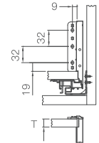
5. Розміри для встановлення задньої стінки Виміри: мм
